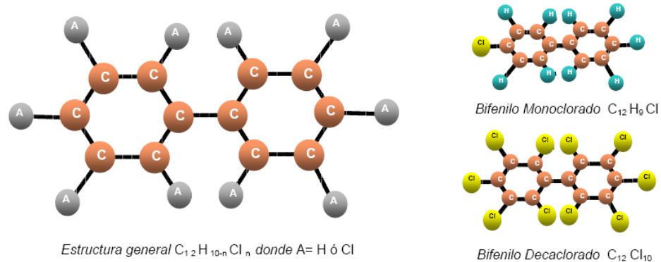
Figura 1. Estructura molecular de los PCB
