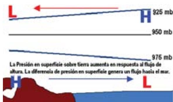
Figura 1-31. Brisa de tierra: desarrollo de alta presión en superficie sobre tierra y de un flujo hacia el mar
