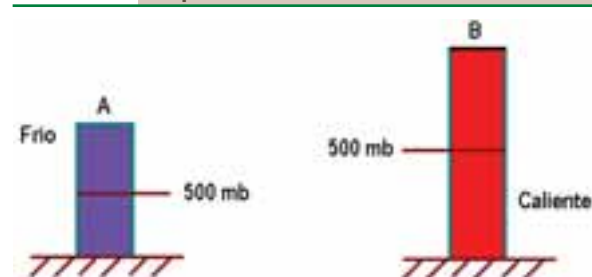
Figura 1-10. Diferencias en altura de superficies de presión atmosférica con distintas temperaturas
