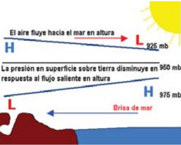
Figura 1-26. Brisa de mar: desarrollo de baja presión en superficie sobre tierra y de un flujo desde el mar hacia la tierra
