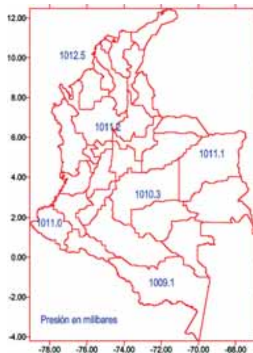
Figura 1-4. Datos de presión reducidos a nivel del mar comunicados por medio de boletines meteorológicos
