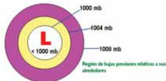
Figura 1-13. Diagrama de un centro de baja presión atmosférica
