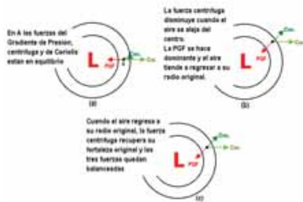
Figura 1-19. Viento Gradiente. Balance de fuerzas: gradiente de presión (PGF), Coriolis (Cor) y Centrífuga (Cen) alrededor de un centro de Baja Presión (L)
