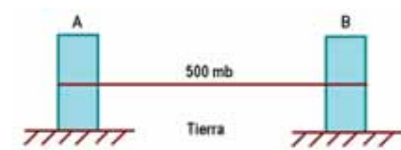
Figura 1-9. Altura de superficies de presión atmosférica con iguales temperaturas
