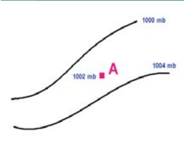
Figura 1-5. Representación gráfica de dos isobaras
