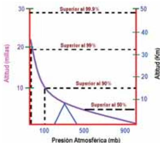
Figura 1-3. Perfil vertical de la presión atmosférica
