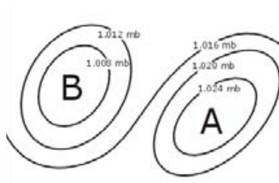
Figura 1-22. Isobaras alrededor de Sistemas de Altas (A) y Bajas (B) presiones.
