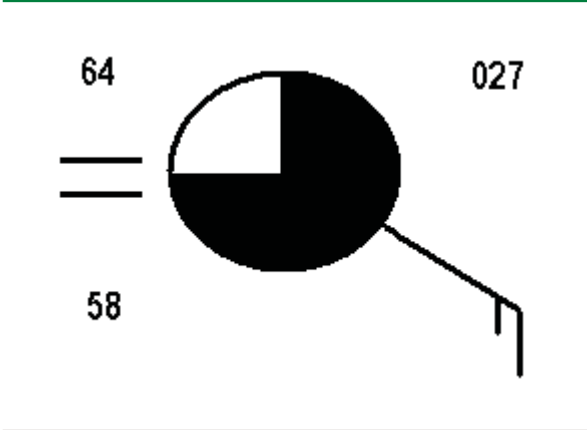
Figura 1-6. Representación gráfica de presión a nivel del mar
