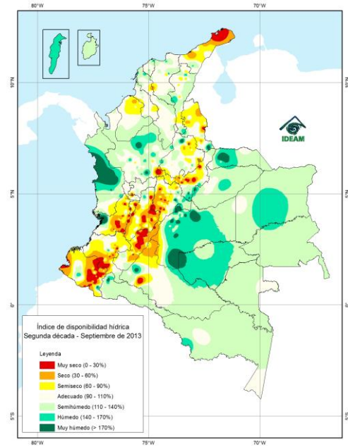
MAPA 8. Disponibilidad hídrica - 2a década
