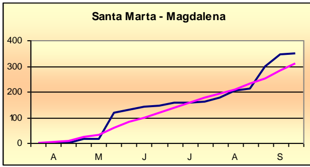
GRÁFICO 9. Precipitación acumulada en los últimos 6 meses a Septiembre 2013
