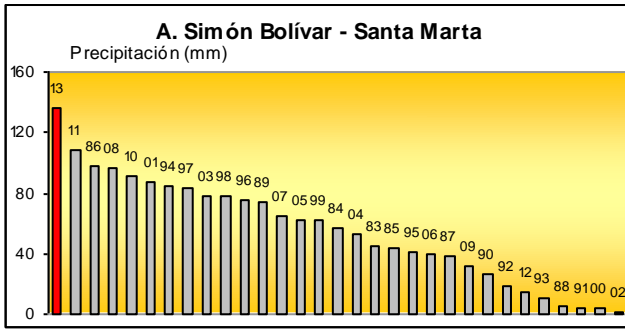
GRÁFICO 1. Precipitación mensual en la perspectiva histórica - Septiembre/2013
