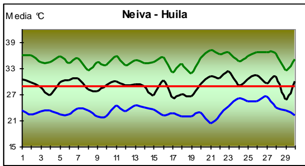
GRÁFICO 13. Seguimiento diario de la temperatura – Septiembre de 2013
