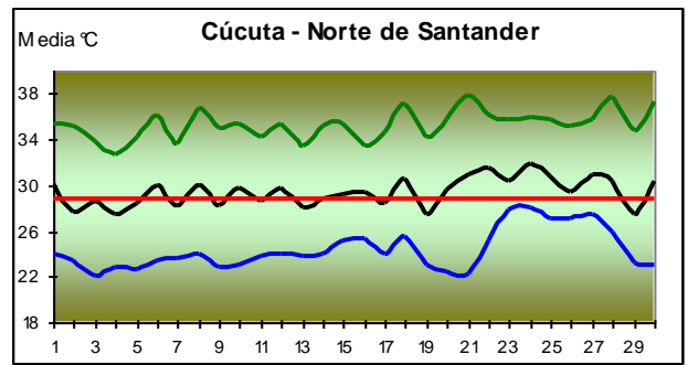
GRÁFICO 12. Seguimiento diario de la temperatura – Septiembre de 2013
