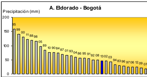
GRÁFICO 2. Precipitación mensual en la perspectiva histórica – Septiembre/2013
