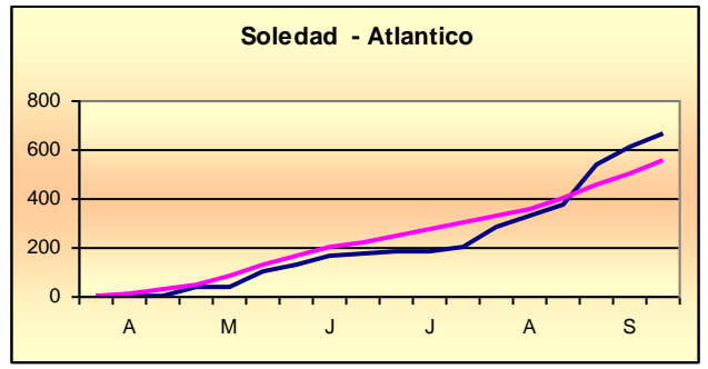
GRÁFICO 9. Precipitación acumulada en los últimos 6 meses a Septiembre 2013
