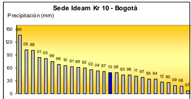
GRÁFICO 2. Precipitación mensual en la perspectiva histórica – Septiembre/2013
