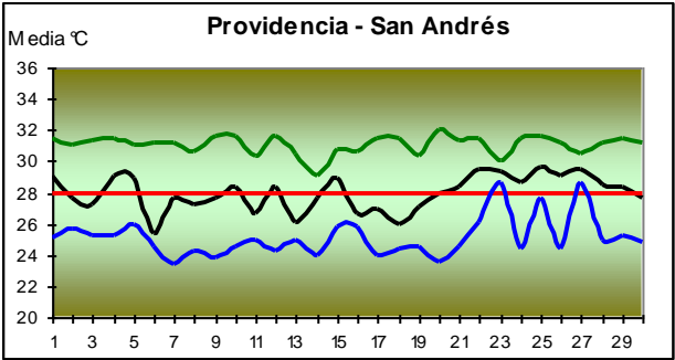
GRÁFICO 11. Seguimiento diario de la temperatura – Septiembre de 2013
