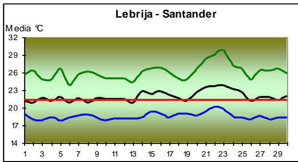
GRÁFICO 12. Seguimiento diario de la temperatura – Septiembre de 2013
