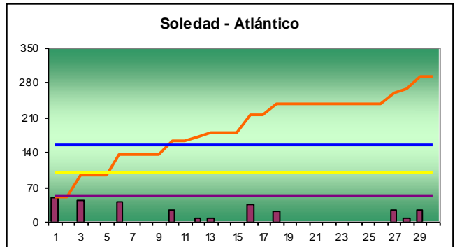
GRÁFICO 4. Seguimiento de la lluvia diaria – Septiembre/2013
