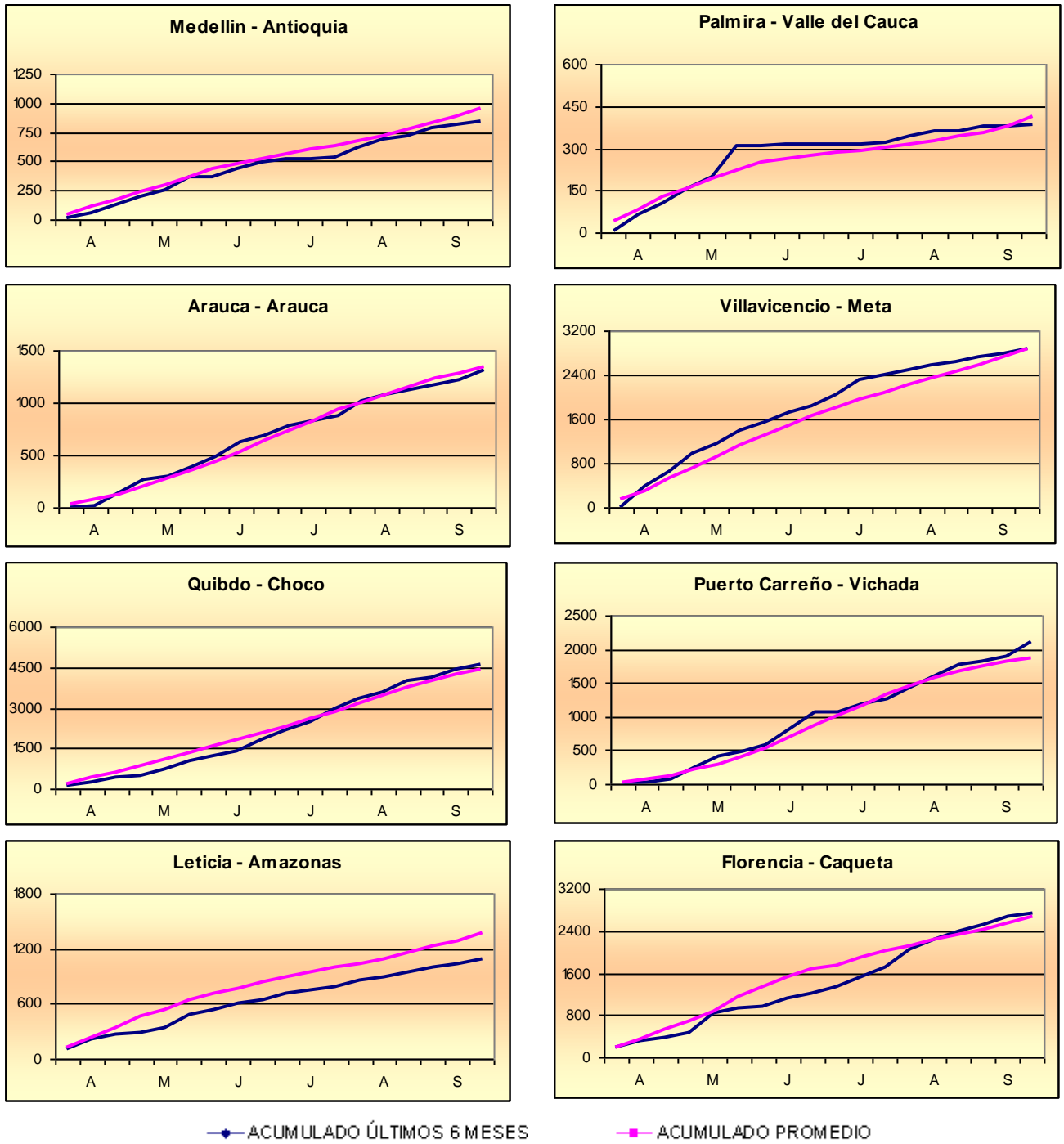
GRÁFICO 10. Precipitación acumulada en los últimos 6 meses a Septiembre 2013
