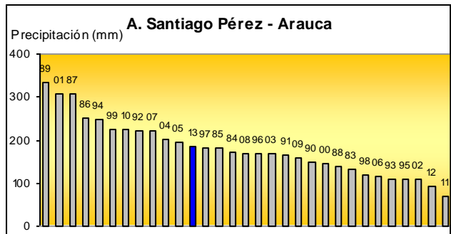
GRÁFICO 3. Precipitación mensual en la perspectiva histórica – Septiembre/2013
