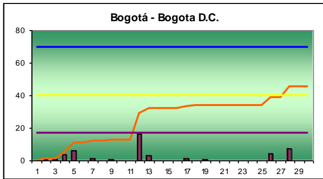
GRÁFICO 5. Seguimiento de la lluvia diaria - Septiembre de 2013
