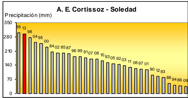
GRÁFICO 1. Precipitación mensual en la perspectiva histórica - Septiembre/2013
