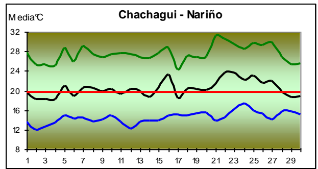
GRÁFICO 13. Seguimiento diario de la temperatura – Septiembre de 2013
