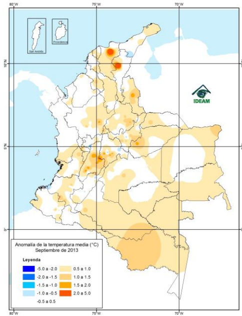
MAPA 4. Anomalía de la temperatura media (°C)
