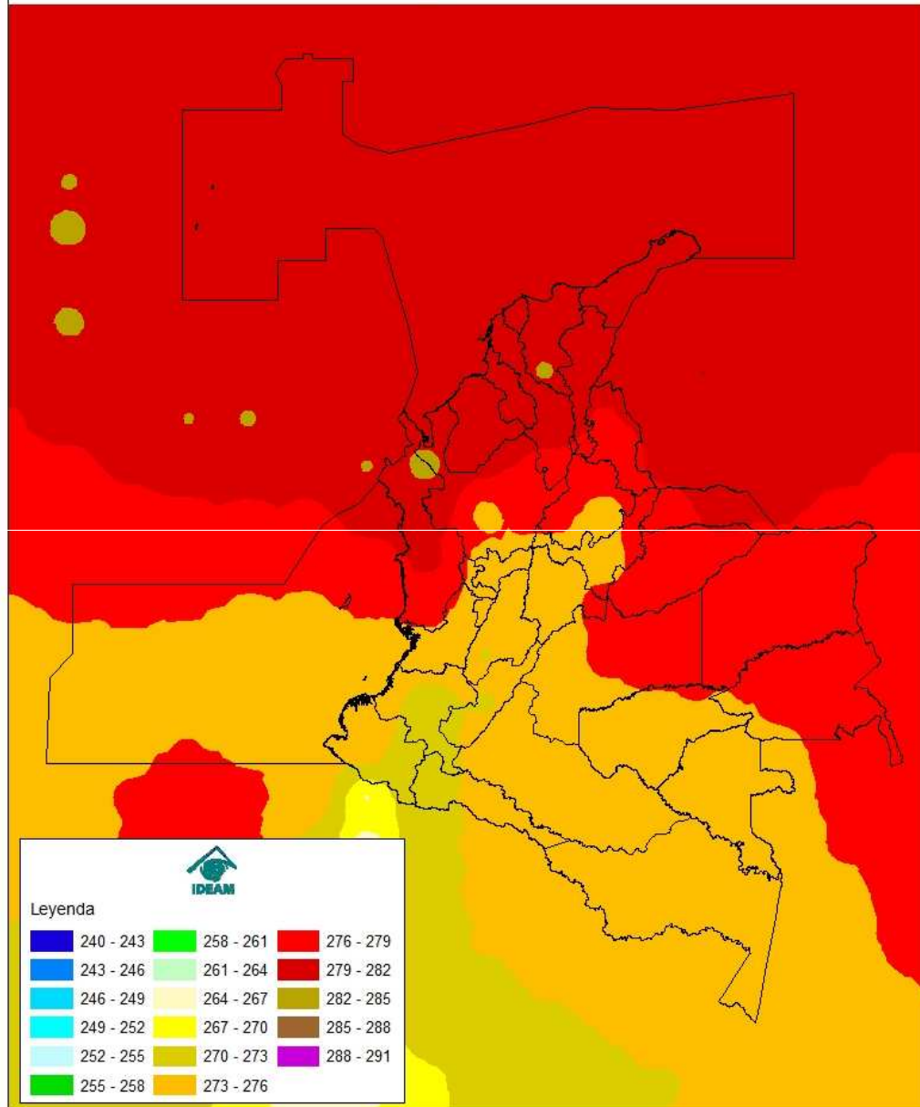
Distribución mensual de la columna de ozono (U.D.) Septiembre
