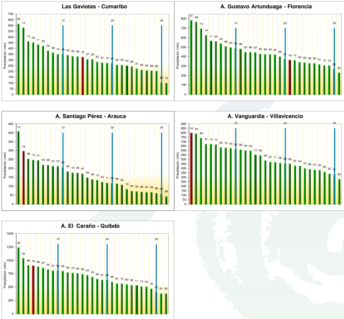
Fig. 9 Número de orden que ocupa el volumen de lluvia mensual actual con relación a los registros de los últimos 30 años.
