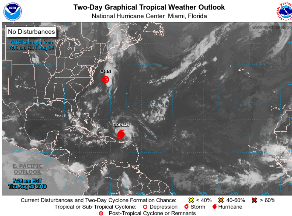
Figura 1 Ubicación huracán DORIAN. Fuente: National Hurricane Center (NHC)
