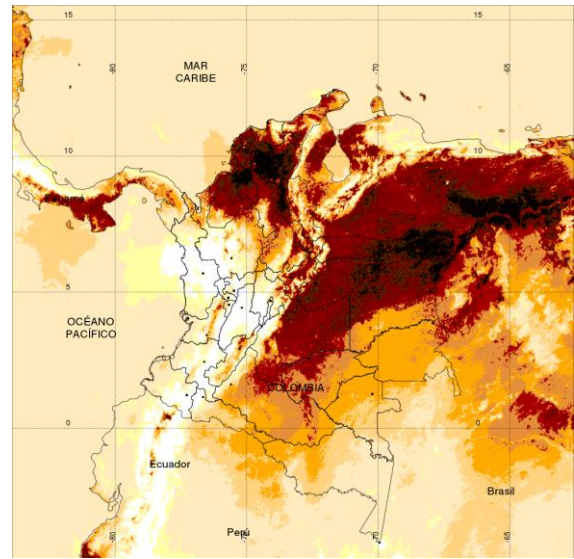
TEMPERATURA SUPERFICIAL MÁXIMA POR ESTIMACIÓN SATELITAL (GOES-16) ( 2019-02-26 09:00:00 a 2019-02-26 18:15:00 ) Elaborado por: Oficina del Servicio de Pronósticos y Alertas. IDEAM INSTITUTO DE HIDROLOGÍA, METEOROLOGÍA Y ESTUDIOS AMBIENTALES
