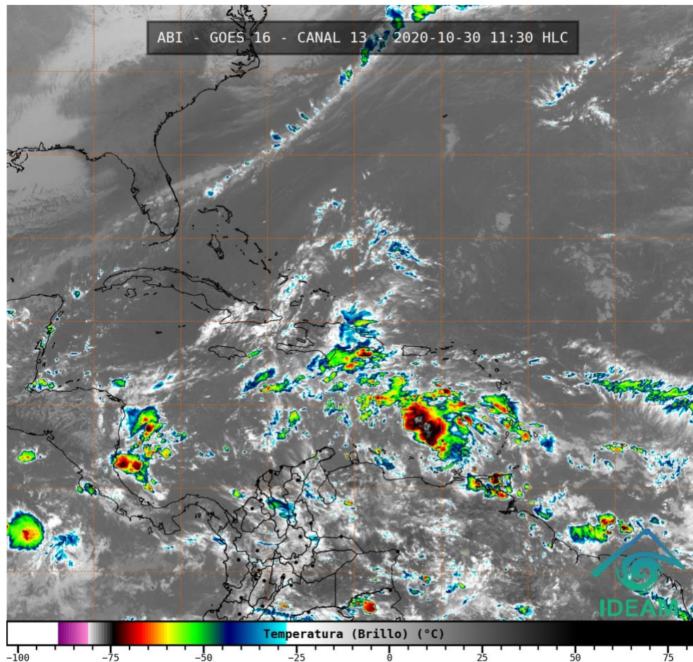
Gráfica 1. Imagen satelital canal infrarrojo GOES – 30 de octubre de 2020. Hora 11:30 HLC.
