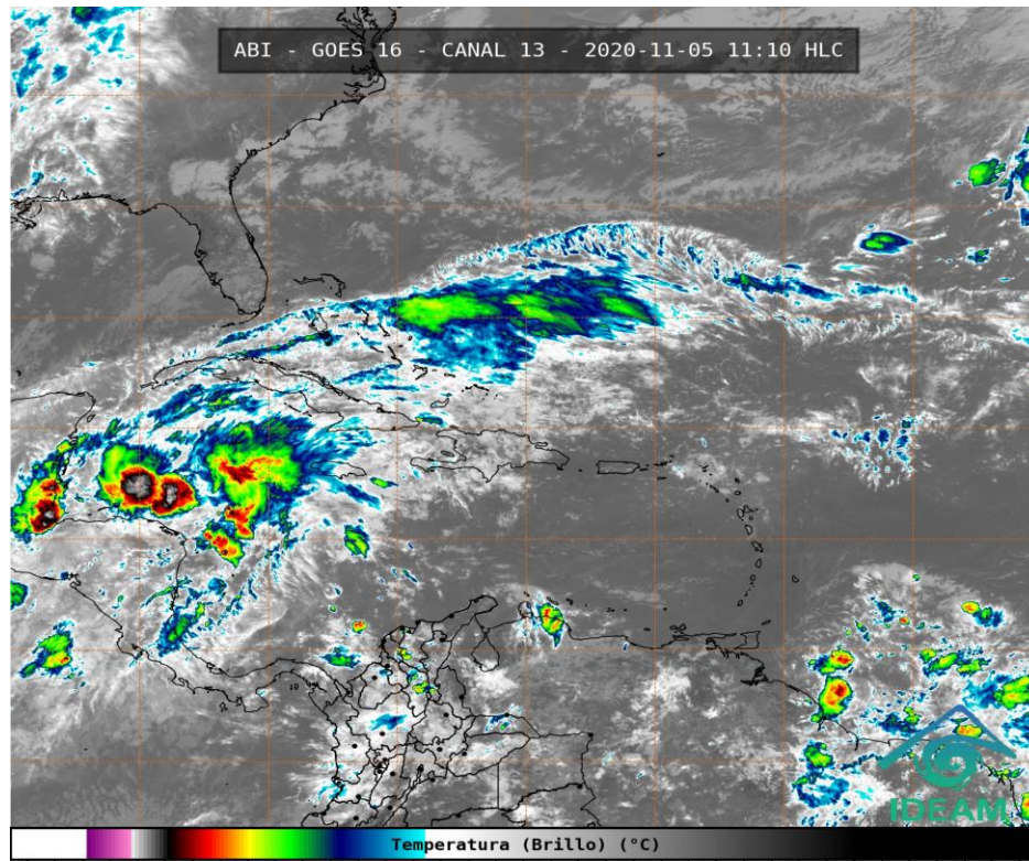
Gráfica 1. Imagen satelital canal infrarrojo GOES 16 – 5 de noviembre de 2020. Hora 11:10 HLC.
