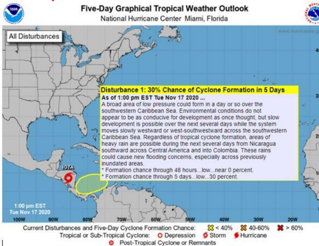
Gráfica 1. Imagen del área donde se observa un 30% de probabilidad de formación ciclónica para los próximos cinco días. Noviembre 17 de 2020. 16:00 HLC. Fuente: NHC-NOAA.
