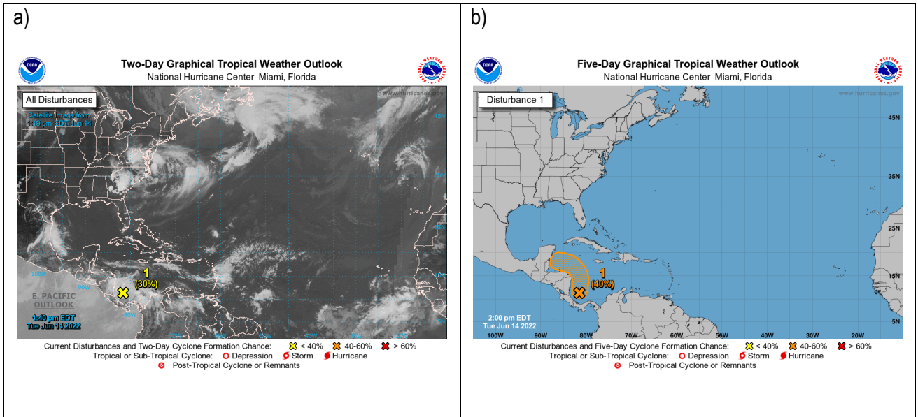
Figura 2. Proyección del Centro Nacional de Huracanes (NHC) 14 de junio de 2022. Hora 12:40 HLC a) Para las próximas 48 horas, y b) Para los próximos 5 días
