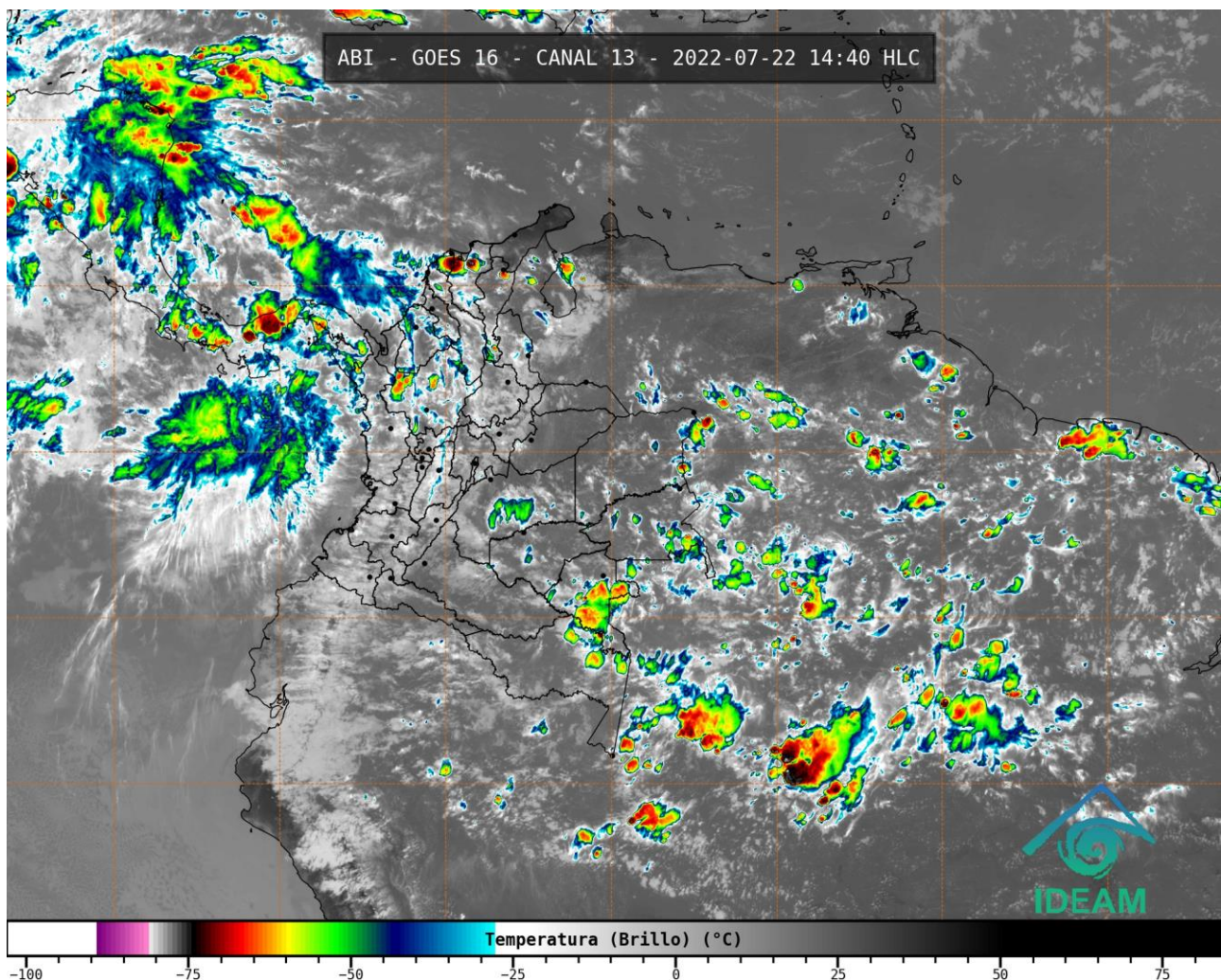
Gráfica 1. Imagen satelital canal infrarrojo GOES - 16, del 22 de julio de 2022. Hora 14:40 HLC.
