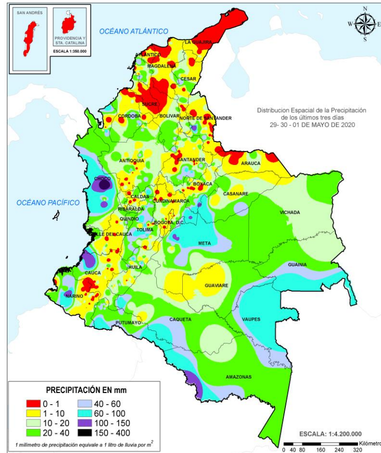
Precipitación últimas 72 horas desde las 7:00 HLC de miércoles 29 de abril hasta las 7:00 HLC del sábado, 2 de mayo de 2020. Fuente: IDEAM
