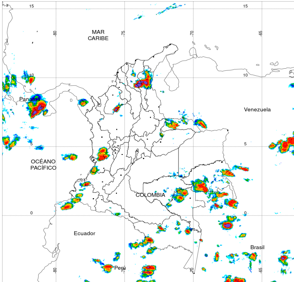
PRECIPITACIÓN TOTAL ACUMULADA POR ESTIMACIÓN SATELITAL (GOES-16) MAY 01 DE 2020 (7:00) - MAY 02 DE 2020 (7:00)
