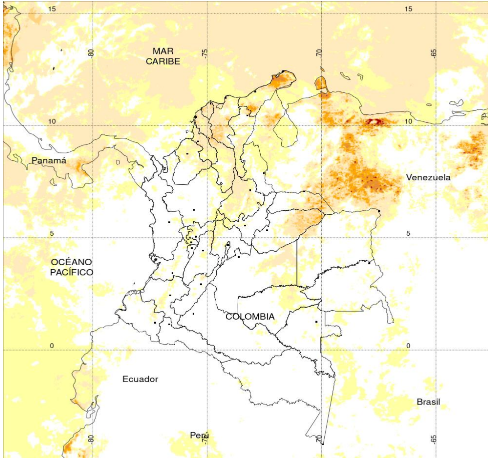
TEMPERATURA SUPERFICIAL MÁXIMA POR ESTIMACIÓN SATELITAL (GOES-16) ( 2020-05-02 09:00:00 a 2020-05-02 09:10:00 )
