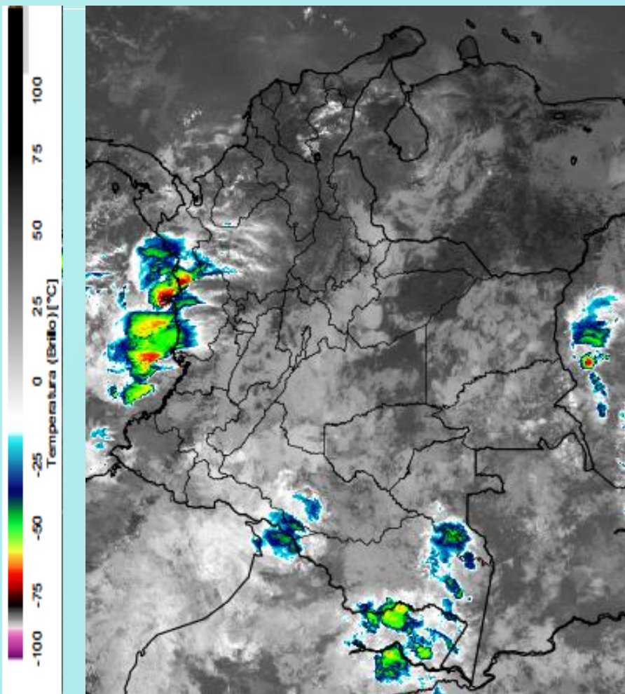
Imagen GOES East Canal Infrarrojo, 2 de mayo de 2020. Hora 9:40 HLC. Fuente: IDEAM-GOES 16
