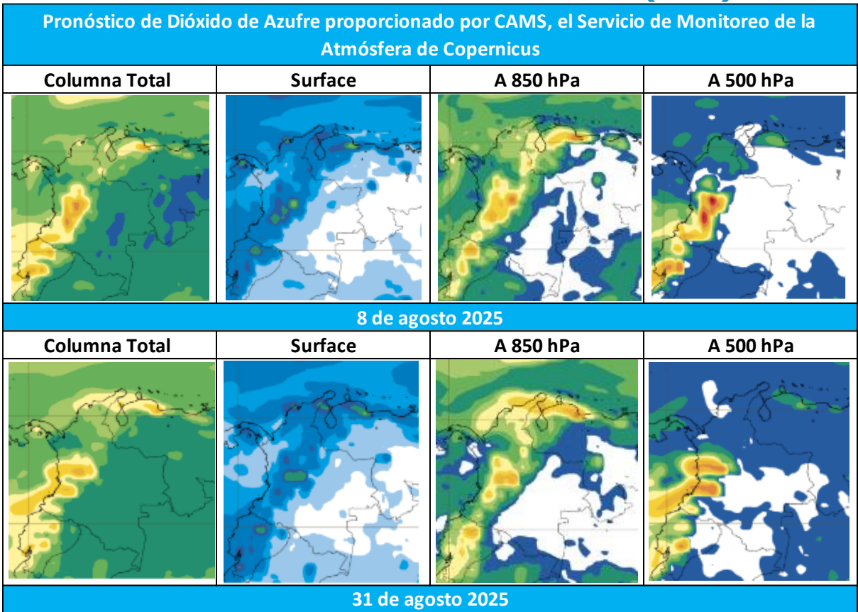
Pronostico dióxido de azufre (SO 2 ). Fuente: proporcionada por CAMS, el Servicio de Monitoreo de la Atmósfera de Copernicus, 2025.
