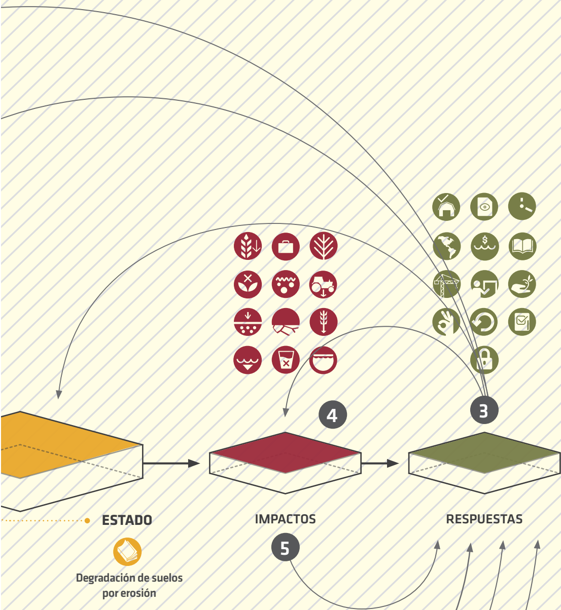
Figura 1.4. ~ Modelo FPEIR o DPSIR. Fuente: Elaboración propia, adoptado de LADA. IDEAM (2014).
