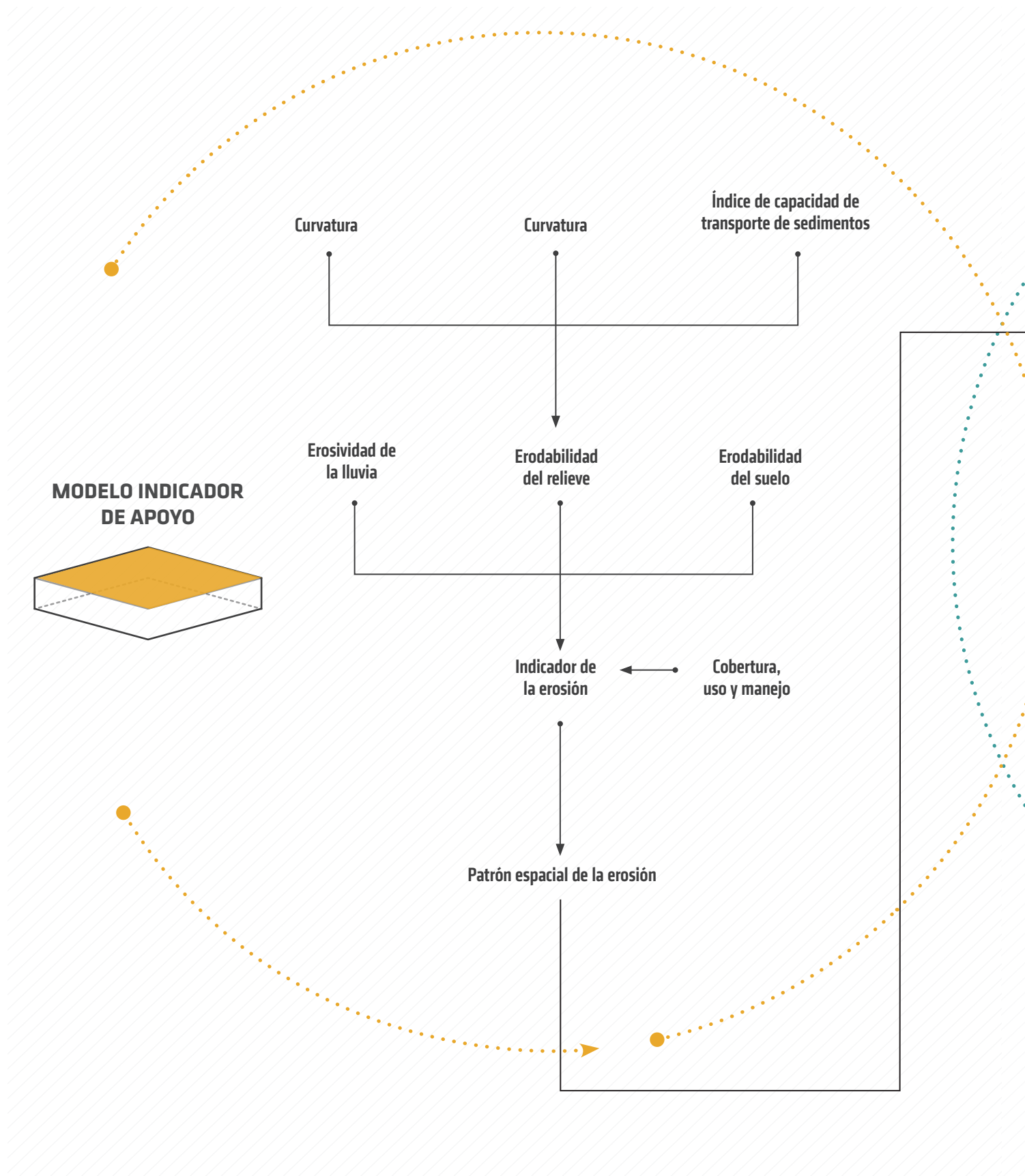
Figura 2.31. ~ Modelo general para elaborar el mapa de zonificación de degradación de suelos por erosión.
