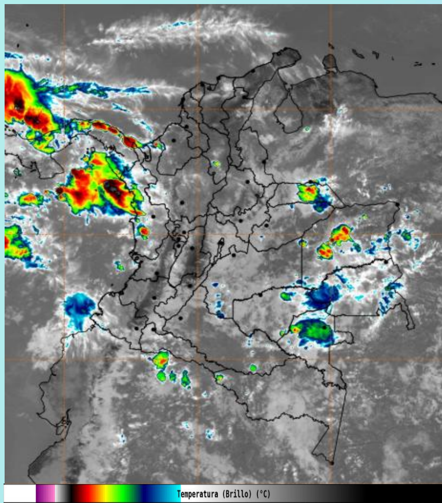
Imagen GOES 19 East Canal Infrarrojo, 22 de julio de 2026 - Hora 11:50 HLC. Fuente: https://bart.ideam.gov.co GOES 19
