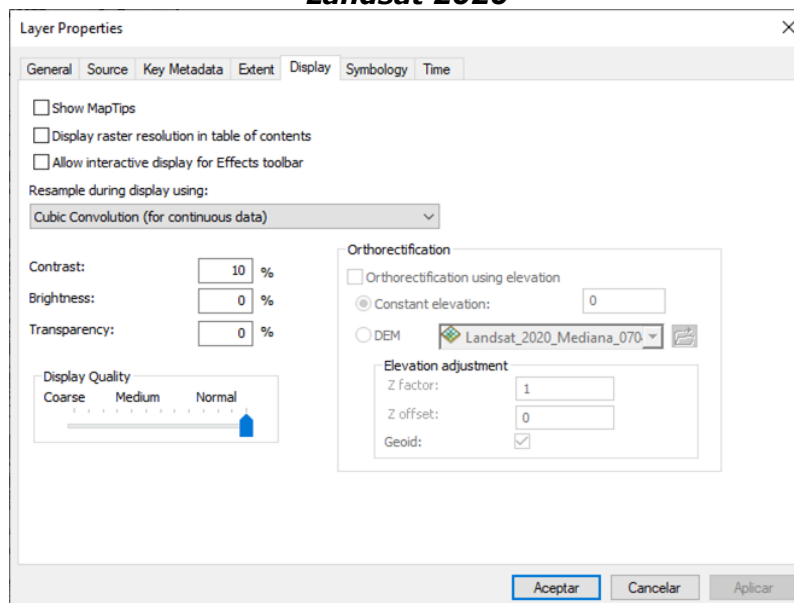
Figura 22 Configuración del remuestreo visual del mosaico medianas Landsat 2020
