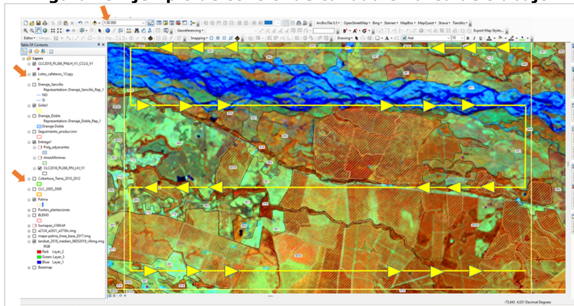
Figura 49 Ejemplo de control de calidad en área de trabajo
