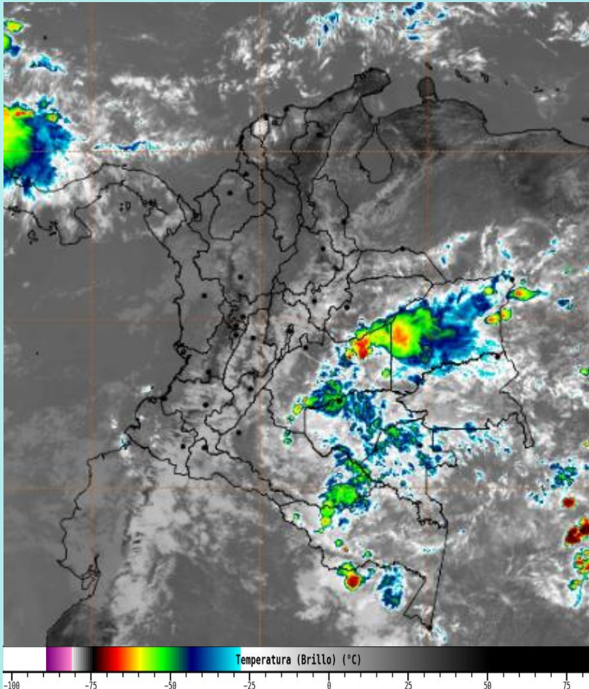
Imagen GOES 19 East Canal Infrarrojo, 07 de agosto de 2026 - Hora 12:00 HLC. Fuente: https://bart.ideam.gov.co GOES 19
