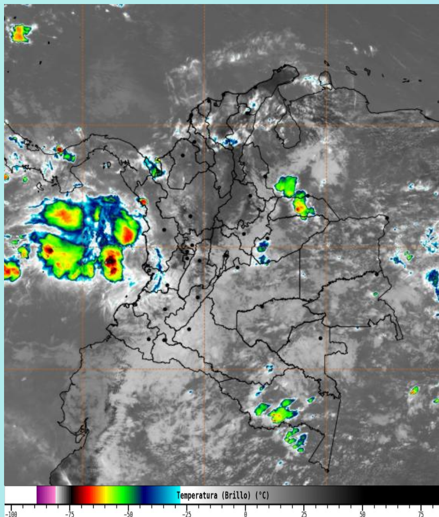
Imagen GOES 19 East Canal Infrarrojo, 14 de agosto de 2026 - Hora 12:00 HLC. Fuente: https://bart.ideam.gov.co GOES 19
