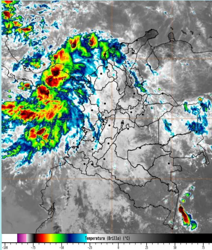
Imagen GOES 19 East Canal Infrarrojo, 17 de agosto de 2026 - Hora 12:10 HLC. Fuente: https://bart.ideam.gov.co GOES 19
