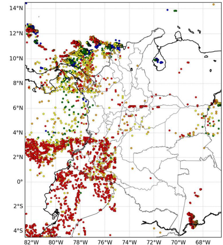
DESCARGAS ELÉCTRICAS GOES 19 MAPA NACIONAL
