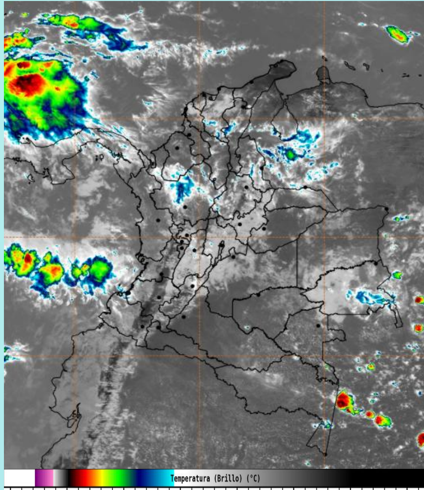
Imagen GOES 19 East Canal Infrarrojo, 01 de septiembre de 2026 - Hora 12:00 HLC. Fuente: https://bart.ideam.gov.co GOES 19
