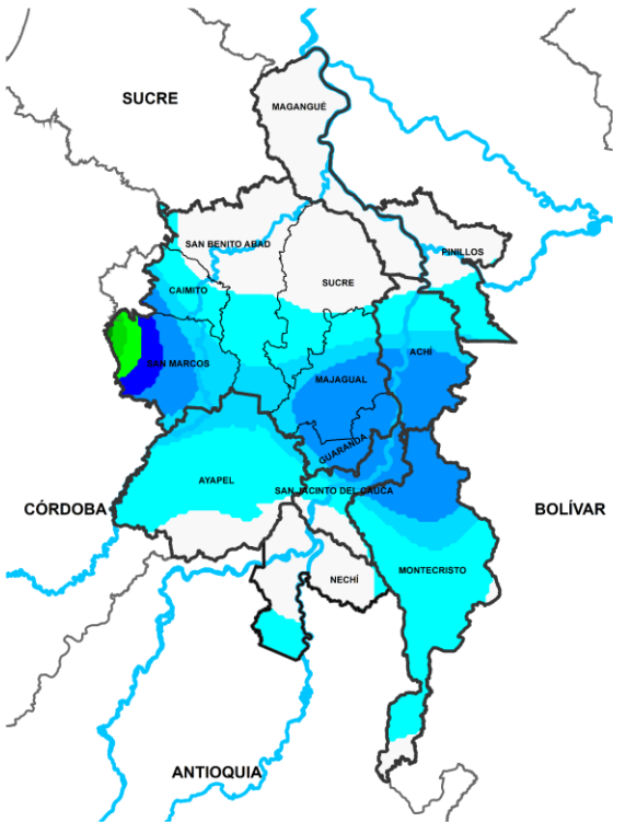
0 0.1 1 2 4 6 8 10 15 20 30 40 60 80 >100 Precipitación Acumulada (mm) Precipitación acumulada 19/02/2026 (07:00) – 20/02/2026 (07:00) Fuente: IDEAM
