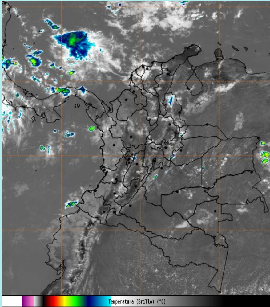
Imagen GOES 19 East Canal Infrarrojo, 05 de octubre de 2026 - Hora 12:00 HLC. Fuente: https://bart.ideam.gov.co GOES 19
