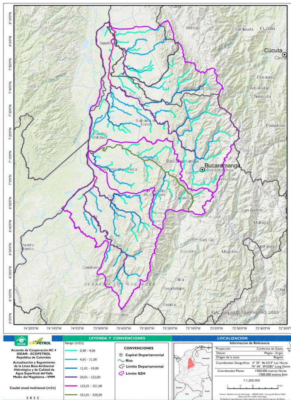
Figura 2.8. Caudal anual multianual en los canales simulados
