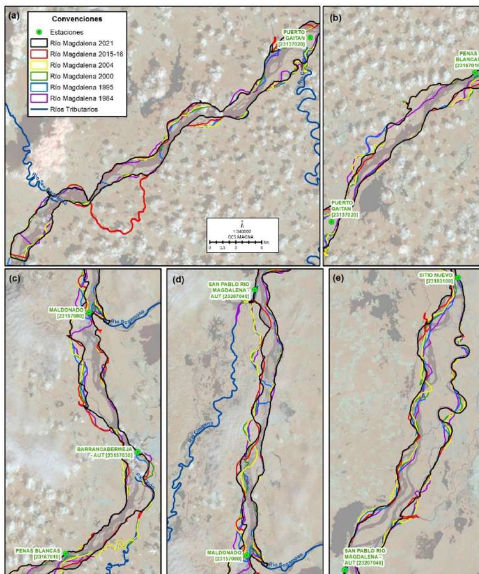
Figura 2.63. Dinámica fluvial del río Magdalena: Puerto Berrío - Sitio Nuevo
