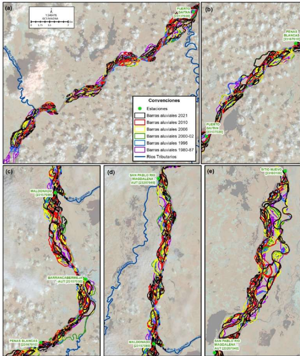
Figura 2.64. Análisis de barras aluviales en el río Magdalena: Puerto Berrío - Sitio Nuevo
