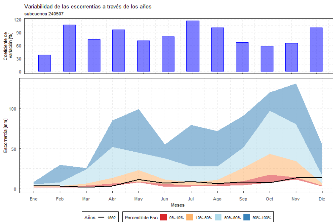
Figura 2.18. Variabilidad interanual de la escorrentía en la unidad de análisis "directos al río Sogamoso, entre Cuchuilla e San Panlo y Marta".
