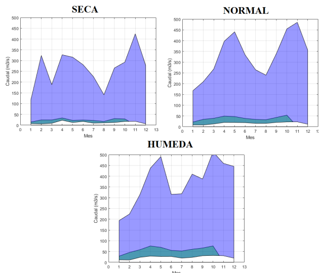
Figura 2. 24. Régimen de caudales antes y después del aprovechamiento máximo para el río La Colorada en el tramo priorizado
