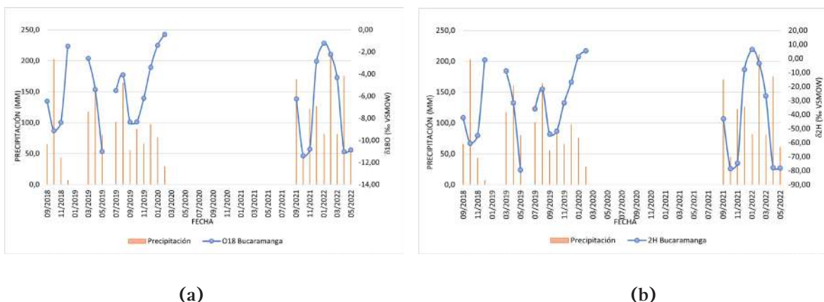
Figura 2.49. Variación temporal de la composición isotópica: (a) \delta^{18}\text{O} y (b) \delta^2\text{H} de la estación de Bucaramanga
