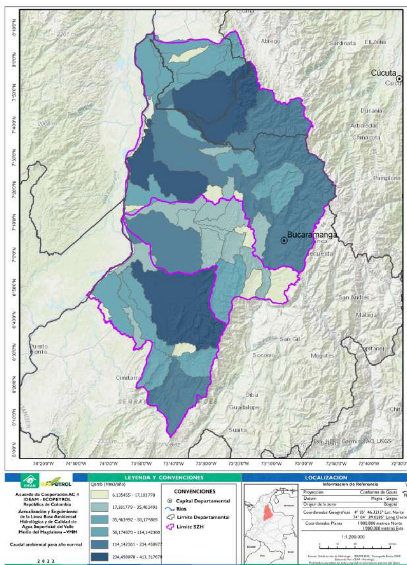
Figura 2. 26. Caudal ambiental calculado con metodología Ideam-ENA para un año normal
