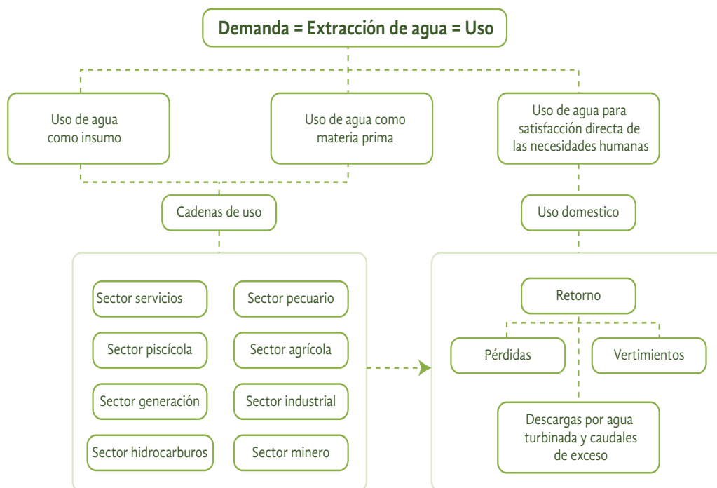
Figura 2.28. Conceptos de demanda hídrica
