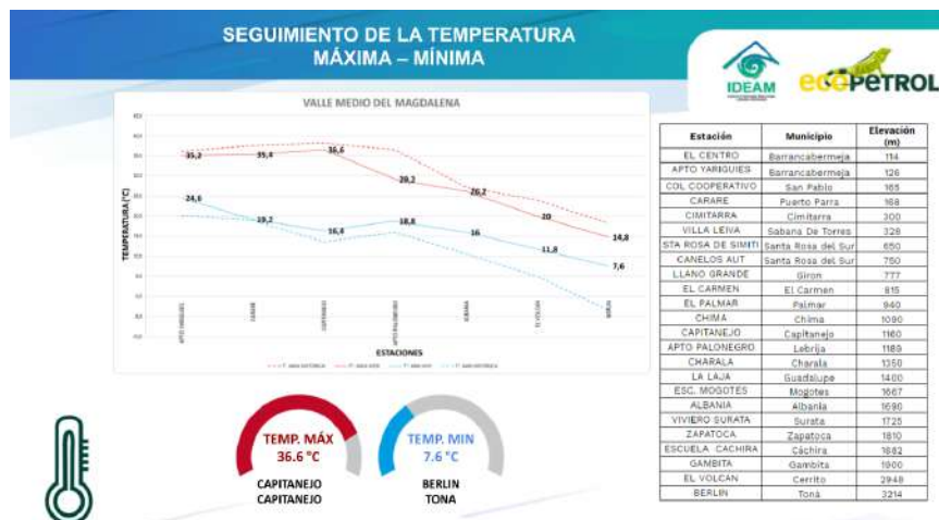
Figura 4.11. Sección del seguimiento a temperaturas máximas y mínimas
