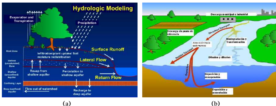
Figura 2. 7. Representación de los procesos hidrológicos en el SWAT. (a) fase terrestre del ciclo hidrológico, (b) fase de tránsito en SWAT
