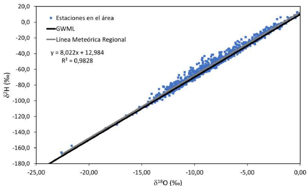
Figura 2.50. Línea meteórica regional de la composición isotópica en el área de interés
