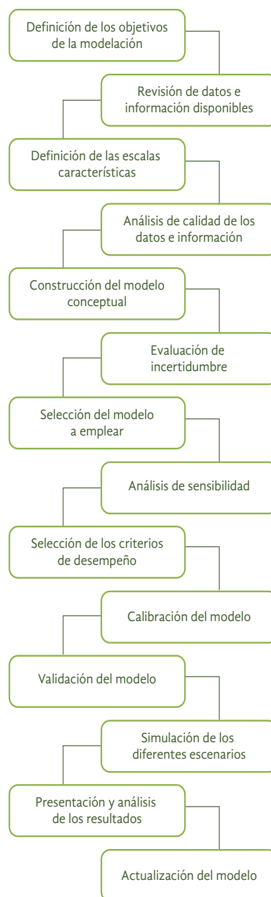
Figura 2. 6. Etapas de la modelación hidrológica
