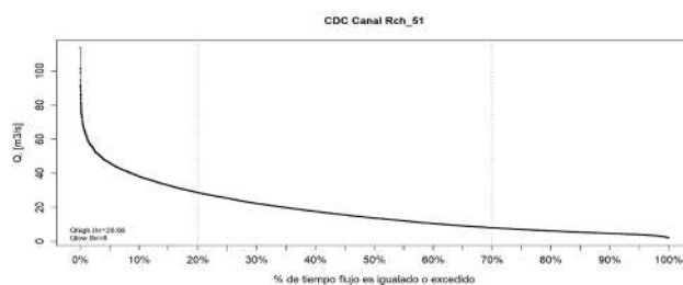
Figura 2.55. CDC diaria de los caudales simulados en la desembocadura del río Cachirí en el río Lebrija
