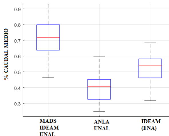
Figura 2. 23. Comparación de los caudales ambientales del río Sogamoso en el sitio de interés con otras metodologías aplicadas en la gestión del recurso hídrico en Colombia
