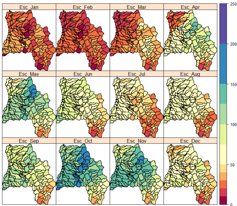
Figura 2. 15. Variación espacial de la escorrentía mensual multianual en milímetros en la SZH del río Lebrija
