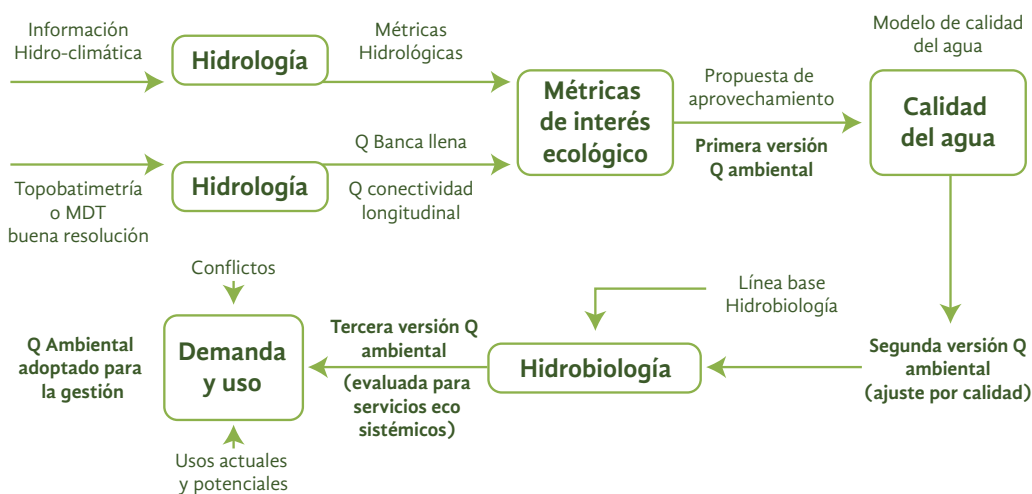
Figura 2. 19. Diagrama de flujo de la aplicación de la metodología para la estimación del caudal ambiental en el río Bogotá
