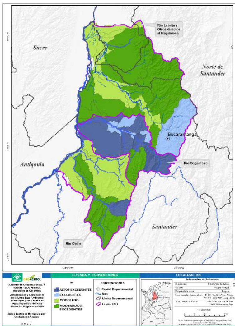
Figura 2.58. Índice de aridez en las unidades de análisis
