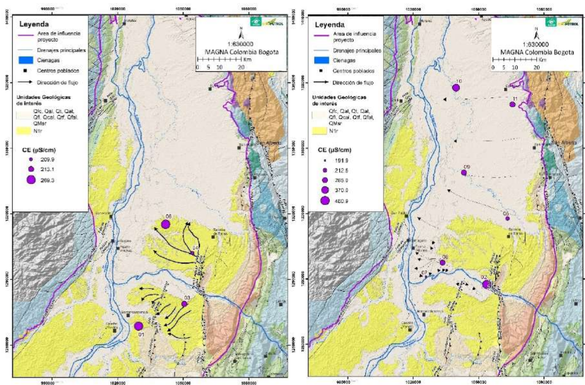
Figura 2.51. Izquierda: mapa de conductividad para puntos que captan el Grupo Real en el sector de Sabana de Torres y al sur del río Sogamoso. Derecha: mapa de conductividad para puntos que captan los Depósitos Cuaternarios en la mayoría del área de influencia
