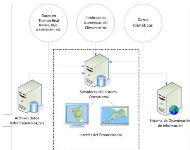
Figura 2.70. Estructura esquemática de un sistema de pronóstico hidrológico y sus enlaces a otros servicios de importancia para el sistema operacional
