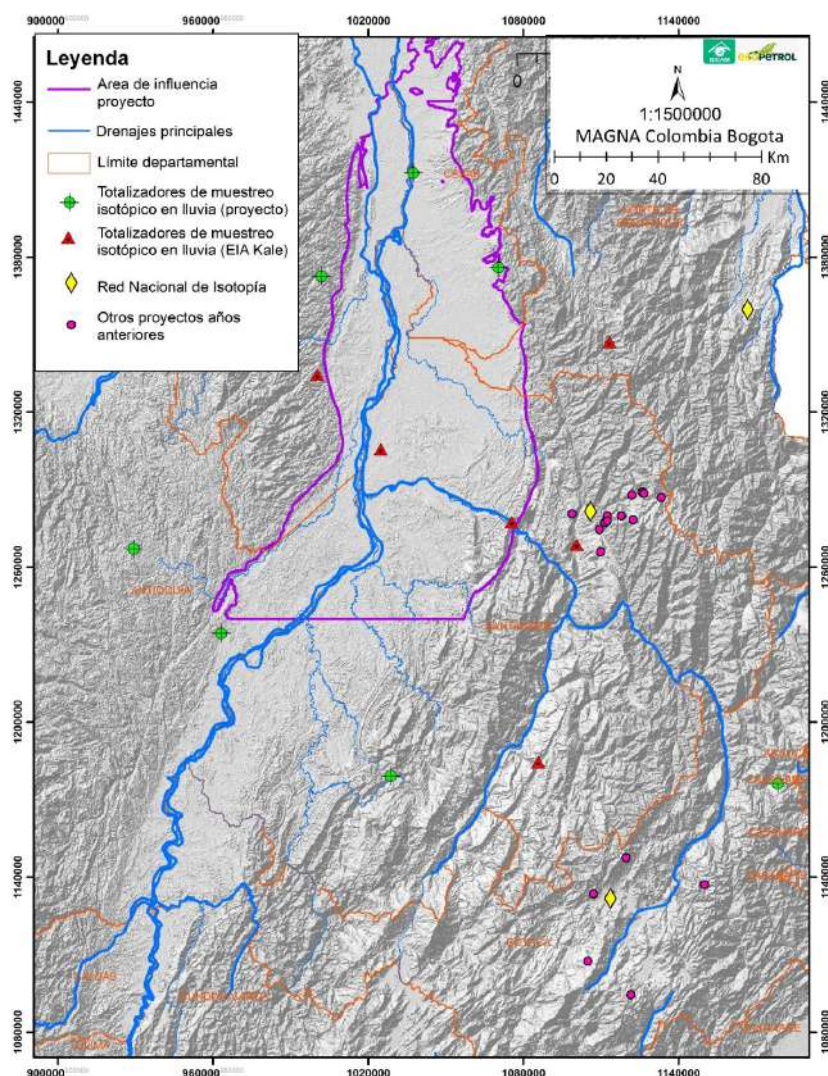
Figura 2.47. Puntos de monitoreo isotópico en agua lluvia considerados para el análisis
