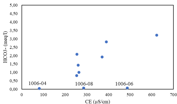
Figura 2.53. Relación entre el \text{HCO}_3^- y la conductividad eléctrica
