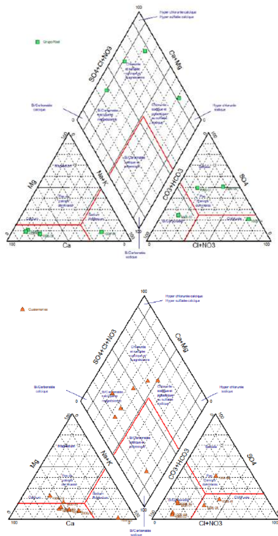
Figura 2.52. Diagrama Piper para las captaciones del Grupo Real y Depósitos Cuaternarios
