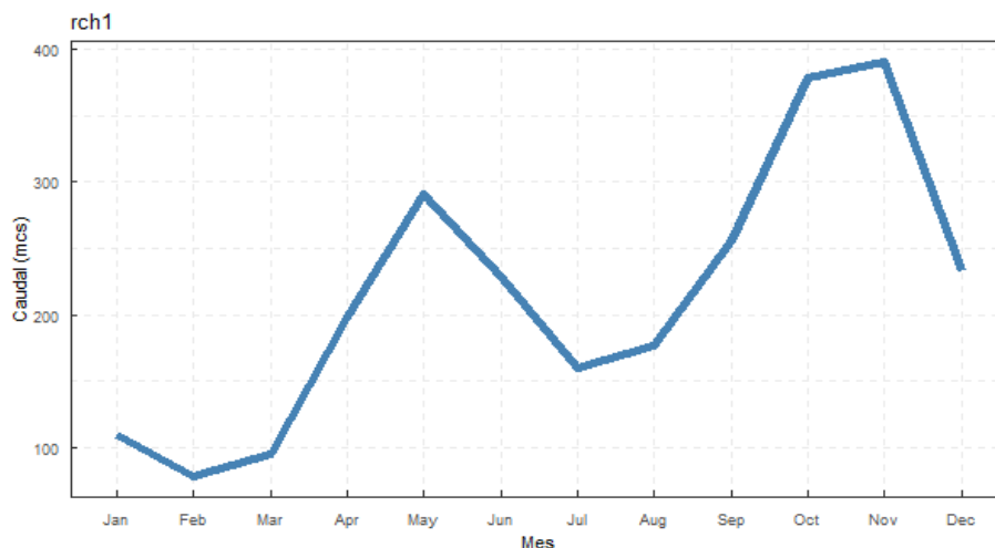
Figura 2. 9. Variación intraanual de los caudales en mcs (metros cúbicos/segundo) para el canal del río Lebrija que desemboca directamente al río Magdalena
