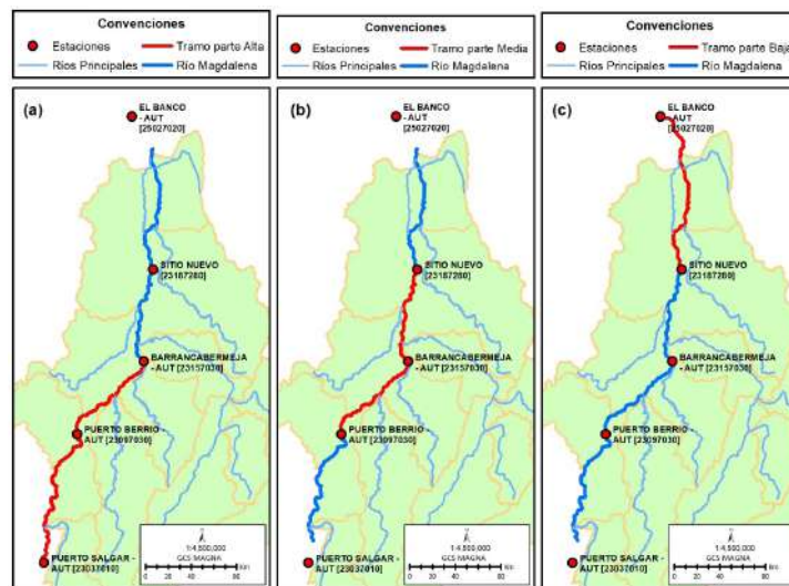
Figura 2.68. Tramos de modelación hidráulica del río Magdalena: (a) parte alta, (b) parte media y (c) parte baja
