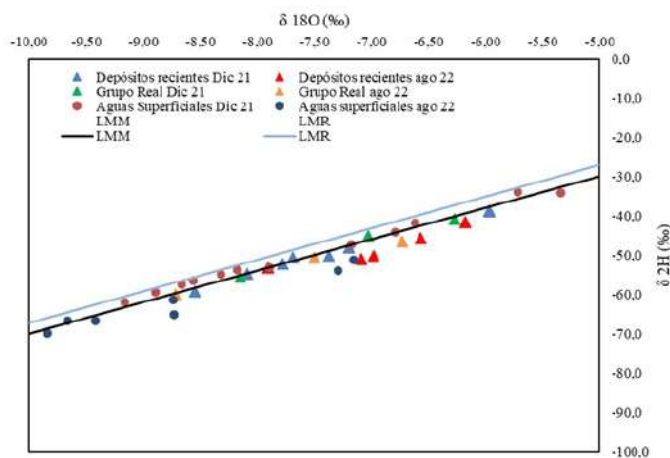
Figura 2.54. Variación de la composición isotópica del agua subterránea y superficial en el Valle Medio del Magdalena respecto a la línea meteórica mundial
