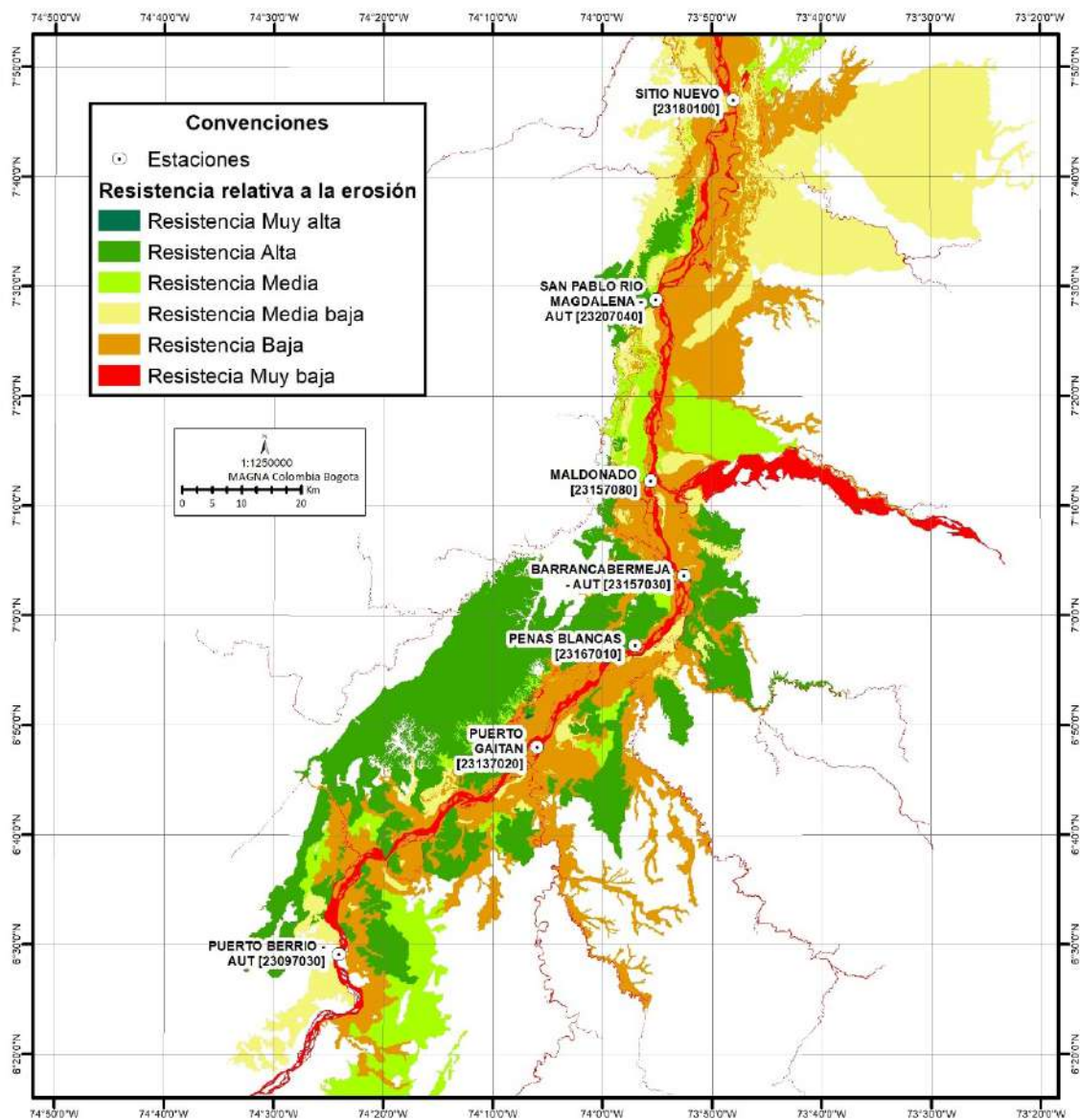
Figura 2.65. Zonificación de la resistencia relativa a la erosión fluvial en el área de interés
