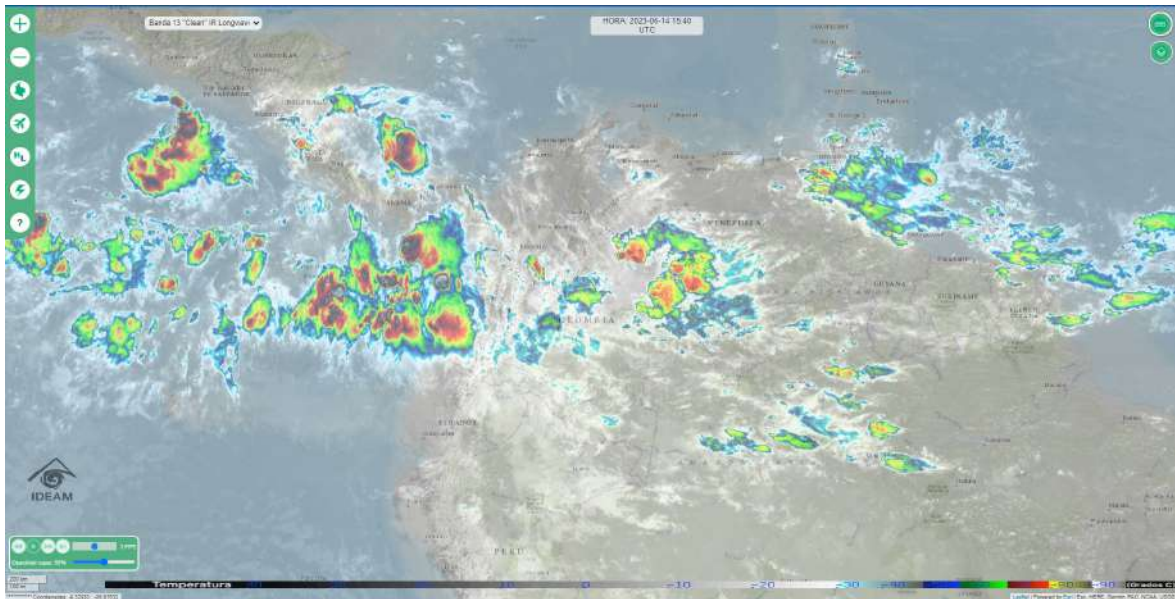
Figura 4. 2. Previsiones de precipitaciones. Imagen canal IR.
