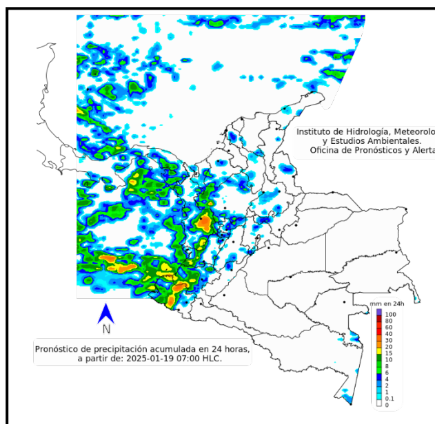
Figura 3 Pronóstico de precipitación acumulada en 24 horas, para el domingo 19 de enero de 2025. Fuente: Ideam.
