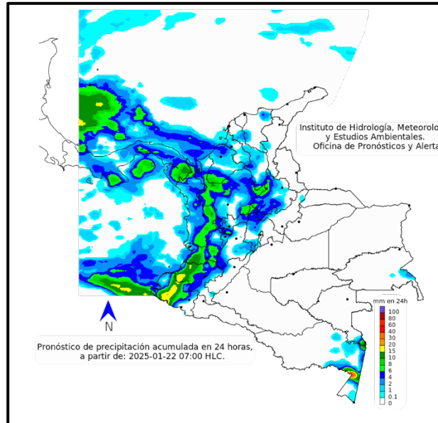
Figura 3 Pronóstico de precipitación acumulada en 24 horas, para el miércoles 22 de enero de 2025. Fuente: Ideam.
