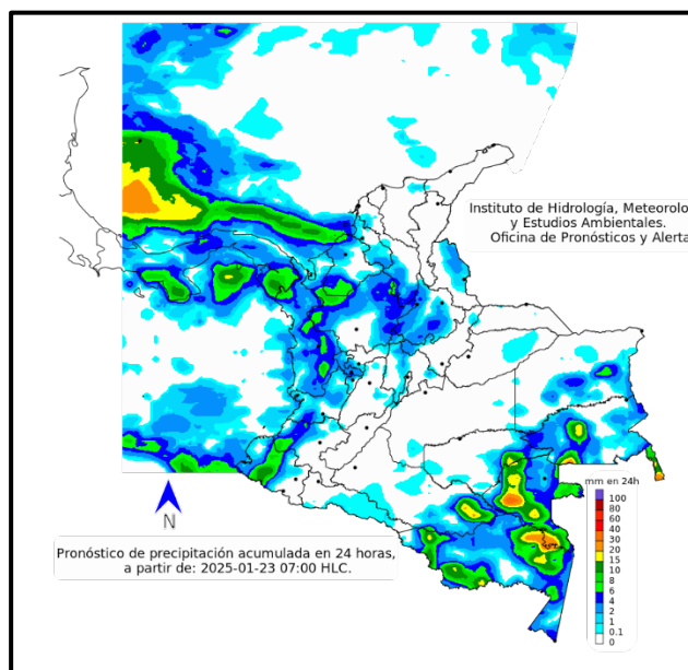
Figura 4 Pronóstico de precipitación acumulada en 24 horas, para el jueves 23 de enero de 2025. Fuente: Ideam.
