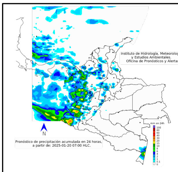
Figura 1. Pronóstico de precipitación acumulada en 24 horas, para el lunes 20 de enero de 2025. Fuente: Ideam.
