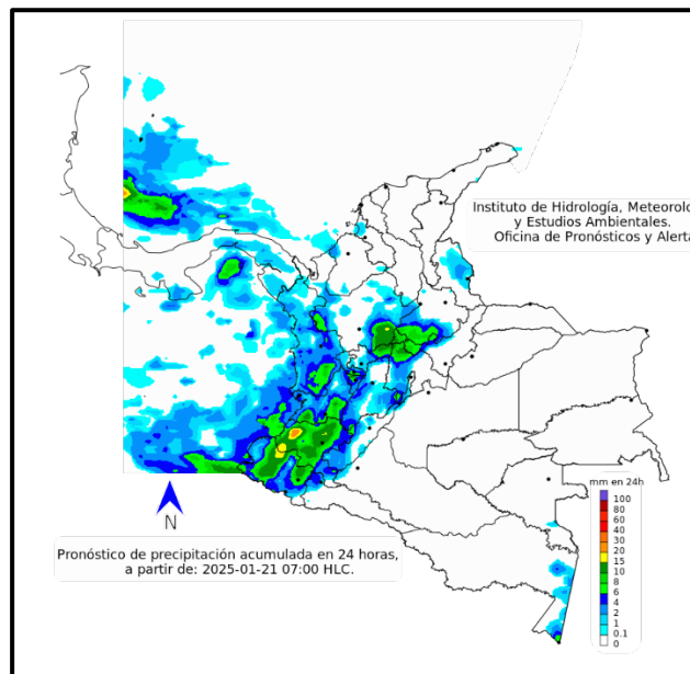
Figura 2. Pronóstico de precipitación acumulada en 24 horas, para el martes 21 de enero de 2025. Fuente: Ideam.
