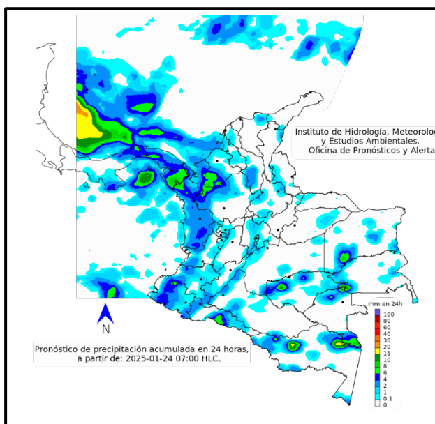
Figura 5 Pronóstico de precipitación acumulada en 24 horas, para el viernes 24 de enero de 2025.
