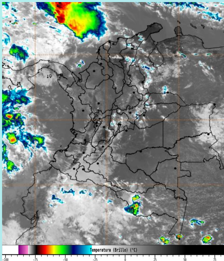
Imagen GOES 19 East Canal Infrarrojo, 24 de julio de 2026 - Hora 12:00 HLC. Fuente: https://bart.ideam.gov.co GOES 19
