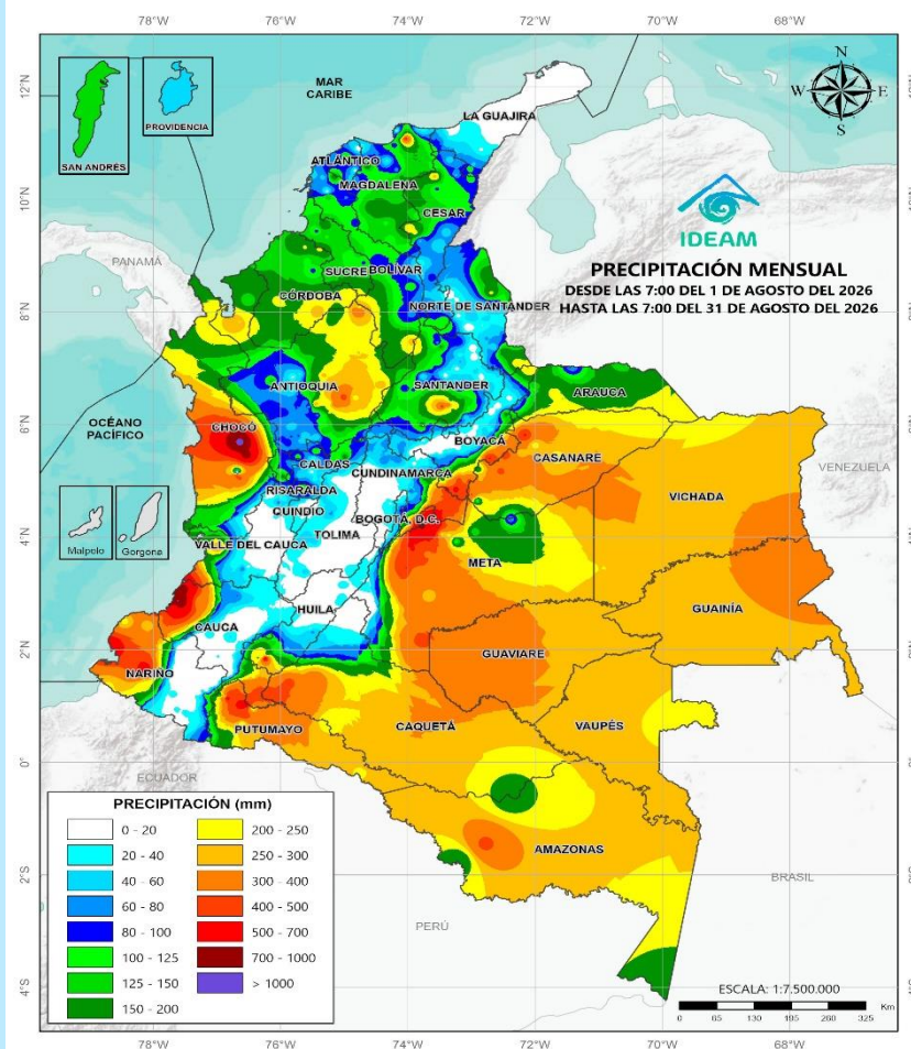
Lluvia acumulada de agosto de 2026
