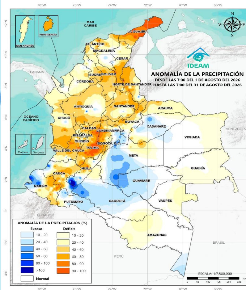
Anomalía ponderada de la lluvia de agosto de 2026
