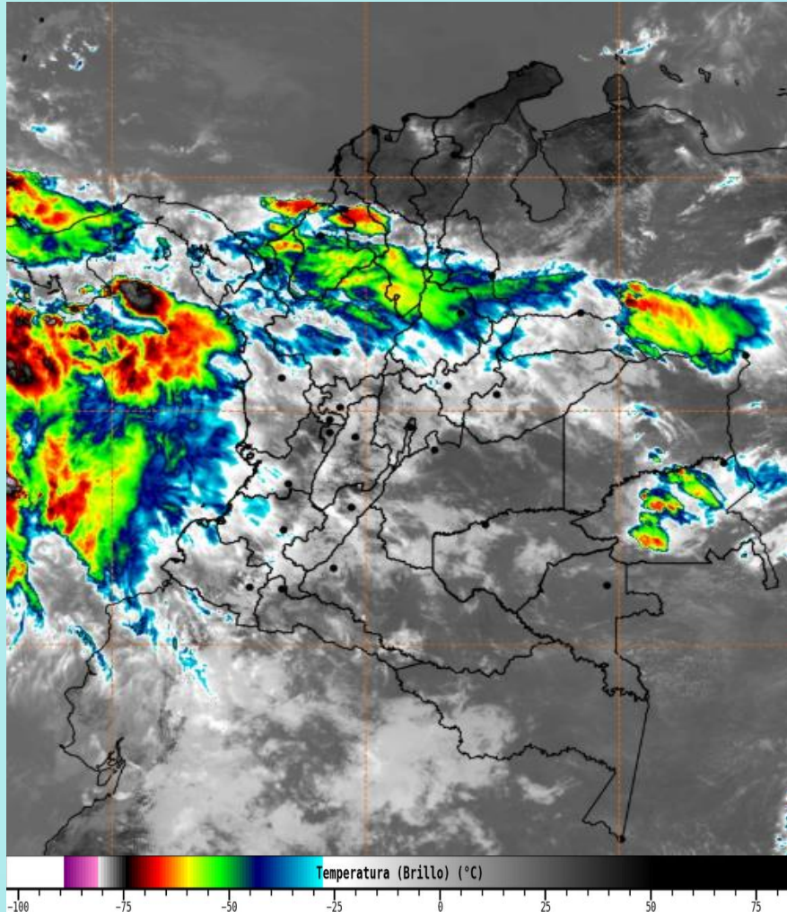
Imagen GOES 19 East Canal Infrarrojo, 06 de septiembre de 2026 - Hora 12:00 HLC. Fuente: https://bart.ideam.gov.co GOES 19
