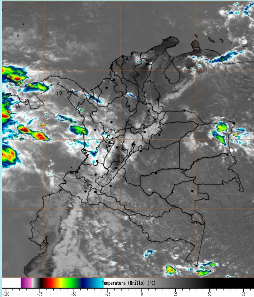
Imagen GOES 19 East Canal Infrarrojo, 01 de agosto de 2026 - Hora 12:20 HLC. Fuente: https://bart.ideam.gov.co GOES 19
