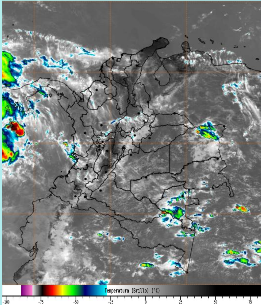
Imagen GOES 19 East Canal Infrarrojo, 02 de agosto de 2026 - Hora 12:00 HLC. Fuente: https://bart.ideam.gov.co GOES 19
