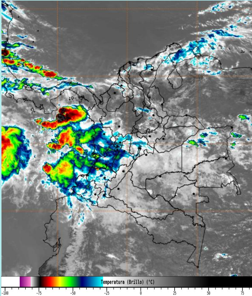
Imagen GOES 19 East Canal Infrarrojo, 05 de agosto de 2026 - Hora 12:00 HLC. Fuente: https://bart.ideam.gov.co GOES 19
