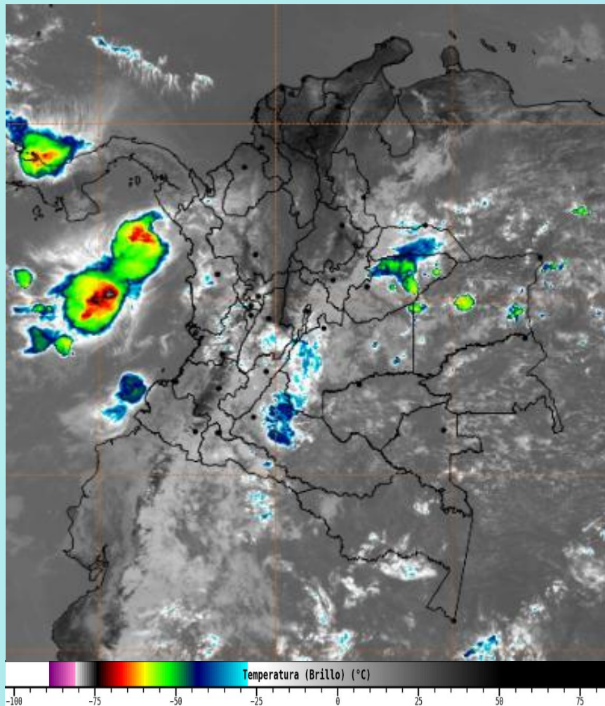
Imagen GOES 19 East Canal Infrarrojo, 08 de agosto de 2026 - Hora 12:00 HLC. Fuente: https://bart.ideam.gov.co GOES 19
