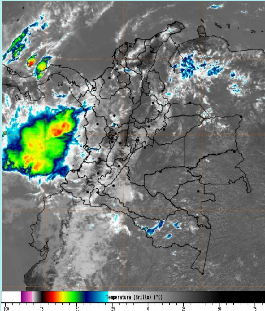
Imagen GOES 19 East Canal Infrarrojo, 09 de agosto de 2026 - Hora 12:00 HLC. Fuente: https://bart.ideam.gov.co GOES 19
