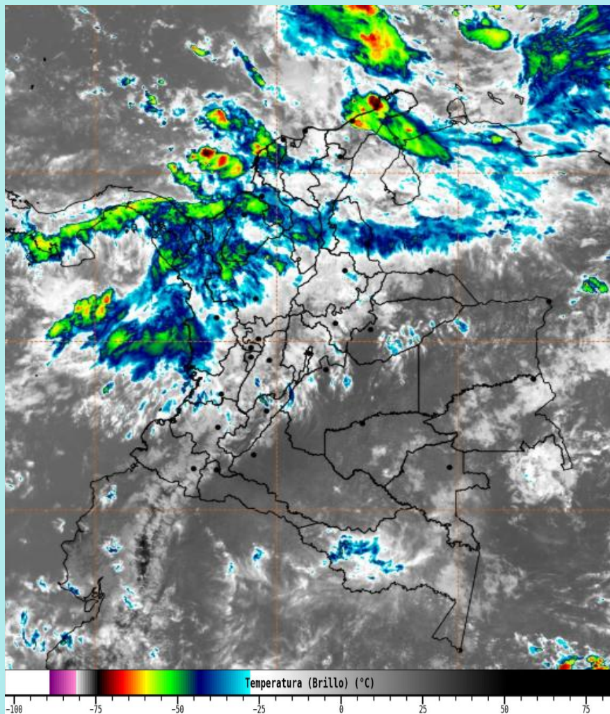
Imagen GOES 19 East Canal Infrarrojo, 13 de octubre de 2026 - Hora 11:50 HLC. Fuente: https://bart.ideam.gov.co GOES 19
